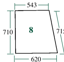
21/4079-1 (D8000/F) Primeros modelos de cabina Early type cab Trasero (superior, fijo) Rear (Upper, fixed)
