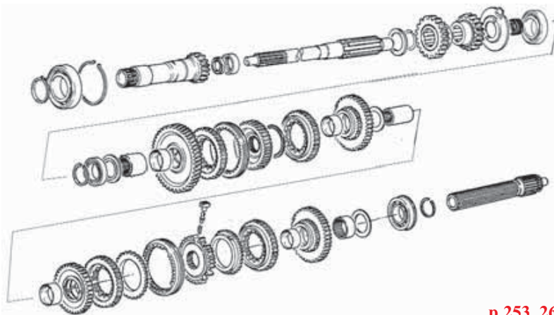
p 253, 267 Arbre primaire / Mainshaft
