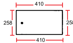
Arrière inférieure / Lower rear
