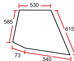
Porte supérieure / Upper door
