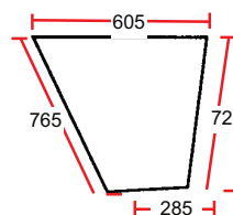
Porte inférieure / Lower door
